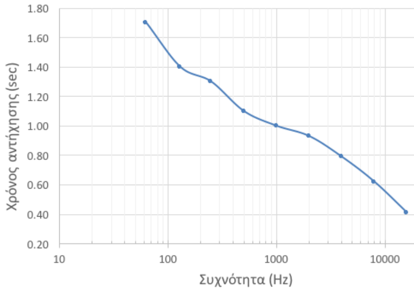
Σχήμα 1. Χρόνος αντίκρισης συναρτήσει της συχνότητας (α) στο χώρο εκδηλώσεων και (β) στο χώρο δημιουργικής απασχόλησης του Αρχοντικού Κουγιουμτζόγλου (Λαογραφικό Μουσείο Ξάνθης).
