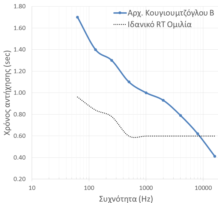
Σχήμα 4. Χρόνος αντήχησης συναρτήσει της συχνότητας στην αίθουσα του Αρχοντικού Κουγιουμτζόγλου (Λαογραφικό Μουσείο Ξάνθης) (α) στο χώρο εκδηλώσεων και (β) στο χώρο δημιουργικής απασχόλησης
