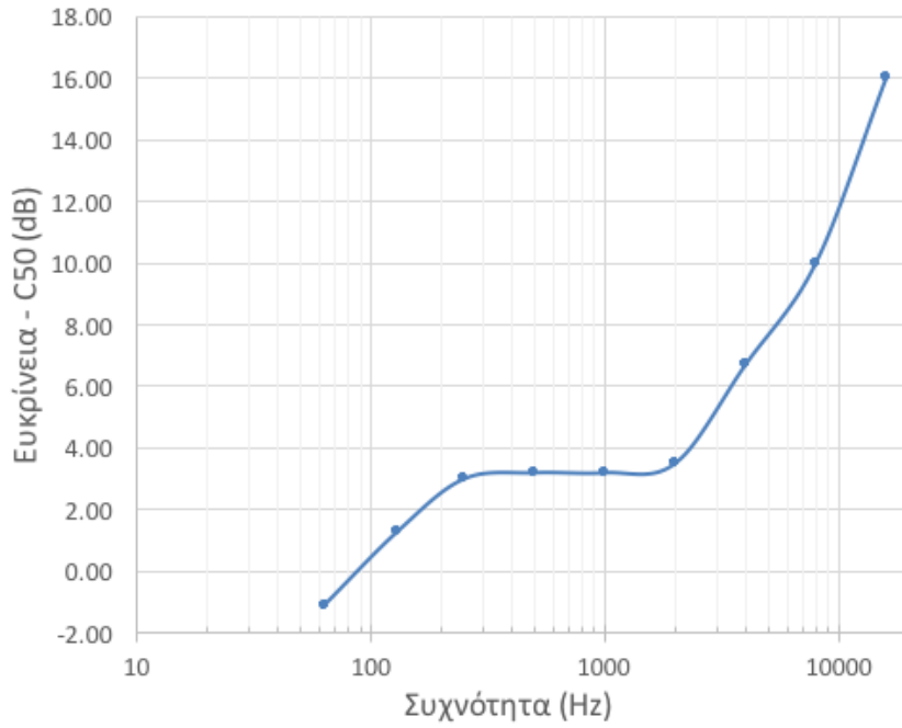
Σχήμα 2. Ακουστική ευκρίνεια (C50) συναρτήσει της συχνότητας (α) στο χώρο εκδηλώσεων και (β) στο χώρο δημιουργικής απασχόλησης του Αρχοντικού Κουγιουμτζόγλου (Λαογραφικό Μουσείο Ξάνθης).
