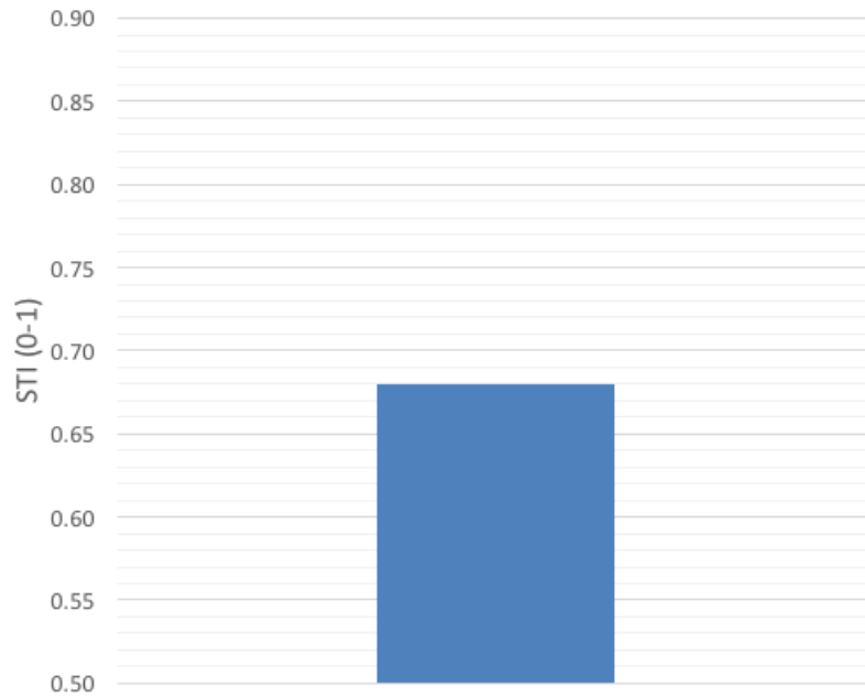
Σχήμα 3 Δείκτης Μετάδοσης Ομιλίας (STI) (α) στο χώρο εκδηλώσεων και (β) στο χώρο δημιουργικής απασχόλησης του Αρχοντικού Κουγιουμτζόγλου (Λαογραφικό Μουσείο Ξάνθης).
